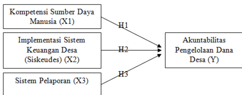
Gambar 1. Desain Penelitian
