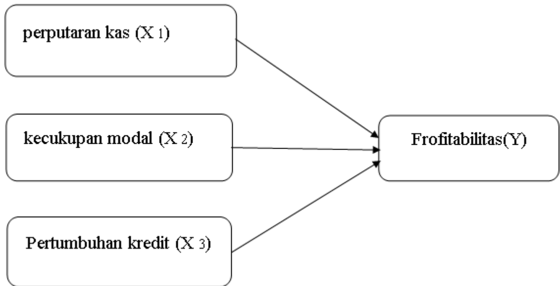
Gambar 1. Kerangka Pemikiran
